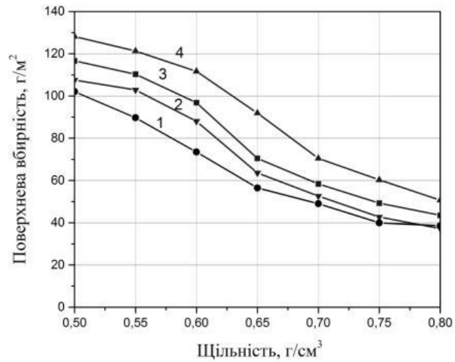
Рис. 2. Залежність поверхневої вбирності від щільності паперу, виготовленого з композиції небіленої сульфатної хвойної і листяної целюлози за різних співвідношень: 1– 100:0; 2 – 80:20; 3 – 70:30; 4 – 60:40
