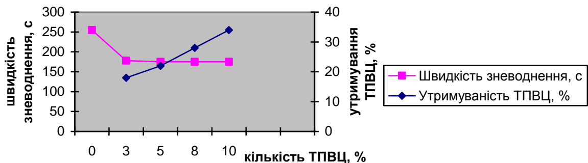
Рис. 1. Зміна технологічних показників паперової маси за різних витрат ТПВЦ
